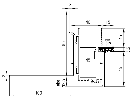
Dimenzije Zeroline dovratnika
