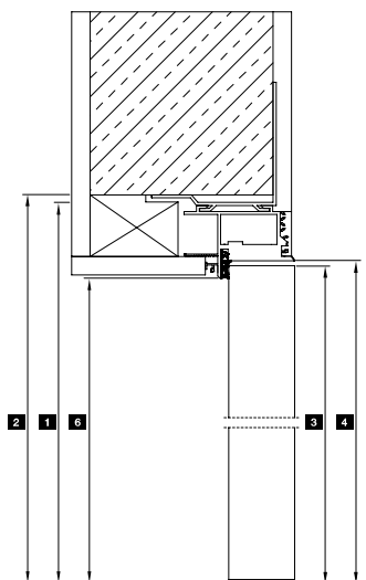
Vertikalni presjek s vratnim krilom u ravni
